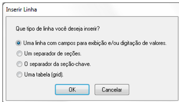
Figura 02 - Adicionando Linha
